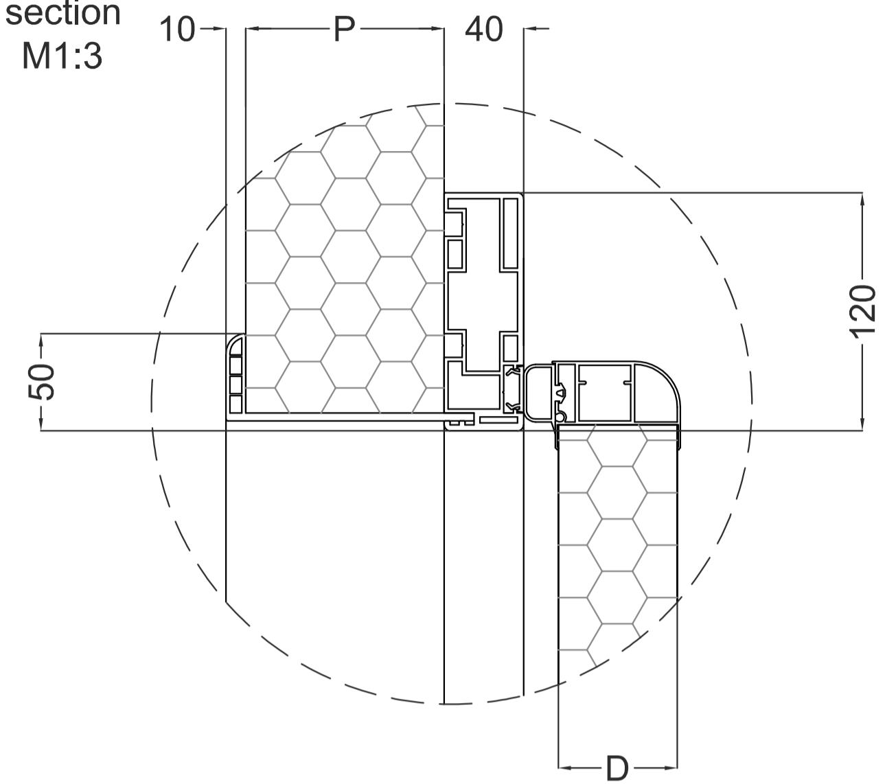
1. Euro2000 ext. lock
